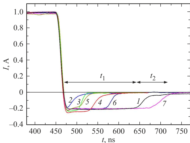
Рис. 2. Осциллограммы переключения p-i-n -диодов с базовыми слоями GaAs (1) и \text{Al}_x\text{Ga}_{1-x}\text{As} с максимальным содержанием x \sim 0.10 (2), 0.2 (3), 0.3 (4), 0.45 (5), 0.6 (6), 0.8 (7). Фазы обратного восстановления t_1 и t_2 указаны для структуры (1).
