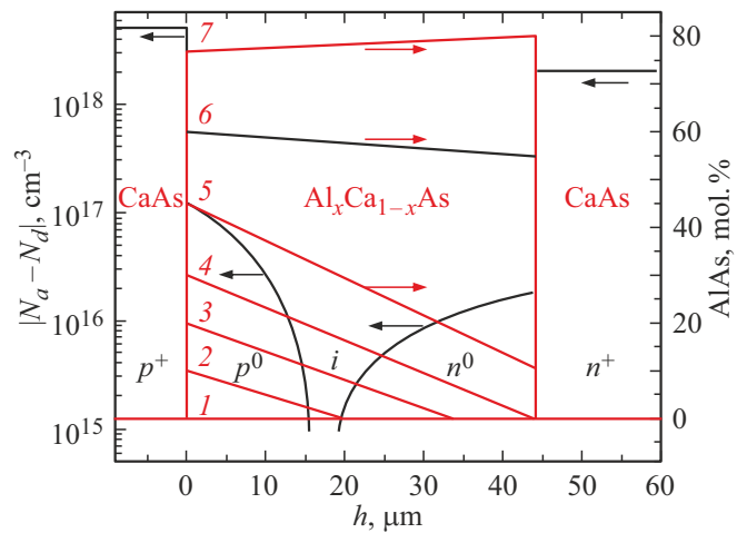
Рис. 1. Распределение свободных носителей заряда |N_a - N_d| (черные линии) по толщине диодных структур p^+-\text{GaAs} (подложка)– \text{Al}_x\text{Ga}_{1-x}\text{As} (плавный p^0-i-n^0 -переход)– n^+-\text{GaAs} (эмиттерный слой). Распределение содержания AlAs (состав x , красные линии) по толщине p-i-n -диодов с базовыми слоями GaAs (1) и \text{Al}_x\text{Ga}_{1-x}\text{As} с максимальным содержанием x \sim 0.10 (2), 0.2 (3), 0.3 (4), 0.45 (5), 0.6 (6), 0.8 (7).
