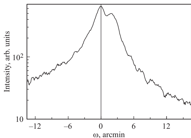
Рис. 2. Кривая качания ( \omega -сканирования) от образца \text{Zn}_{0.99}\text{Mn}_{0.01}\text{Se} , отвечающая рефлексу \text{ZnSe} 220.
