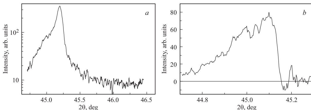
Рис. 1. a — участок рентгеновской дифрактограммы образца \text{Zn}_{0.99}\text{Mn}_{0.01}\text{Se} в окрестности рефлекса \text{ZnSe} 220; b — та же кривая после вычитания модельного пика \text{ZnSe} 220.
