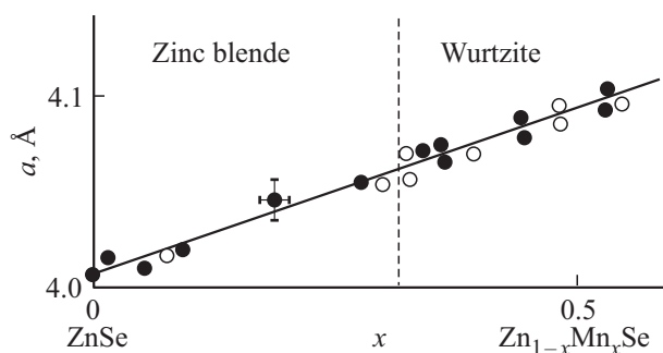
Рис. 3. Сведения о параметрах решетки для различных соединений \text{Zn}_{1-x}\text{Mn}_x\text{Se} , основанные на статье [13] (см. Fig. 1 в работе [13]). По горизонтальной оси (абсцисс) отложена величина, x , характеризующая стехиометрию материала, по вертикальной (ординат) — параметр решетки в Å. Кружки обозначают экспериментальные значения (темные — от порошков, светлые — от монокристаллов), прямая линия — аппроксимацию Вегарда.
