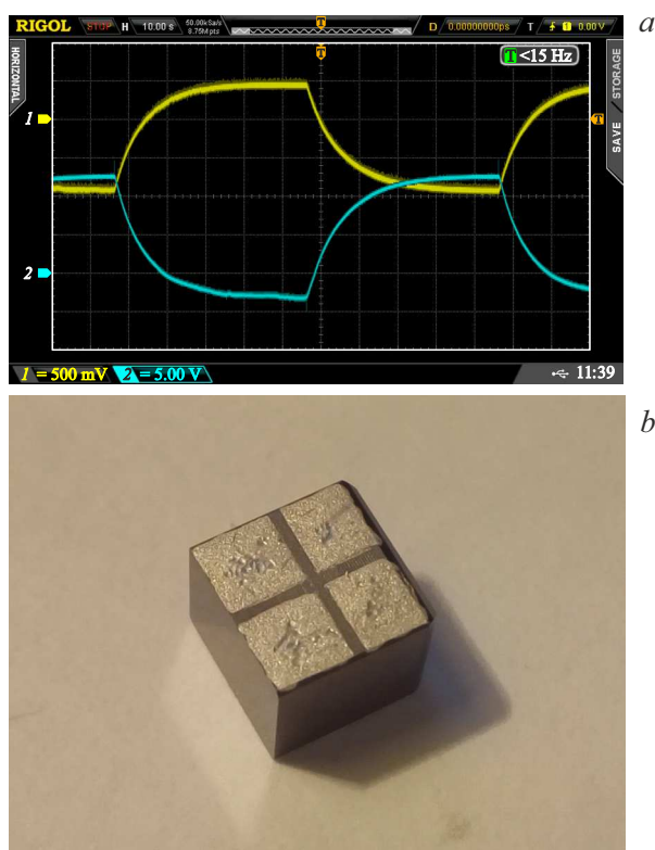
Рис. 3. a — осциллограммы термоэдс дифференциальной медно-константановой термопары (канал 1, желтая линия) и термоэдс кристалла \text{ZnGeP}_2 (канал 2, голубая линия). В обоих каналах используются инструментальные предусилители с коэффициентом усиления 1000. b — образец \text{ZnGeP}_2 с электродами в виде матрицы 2 \times 2 .
