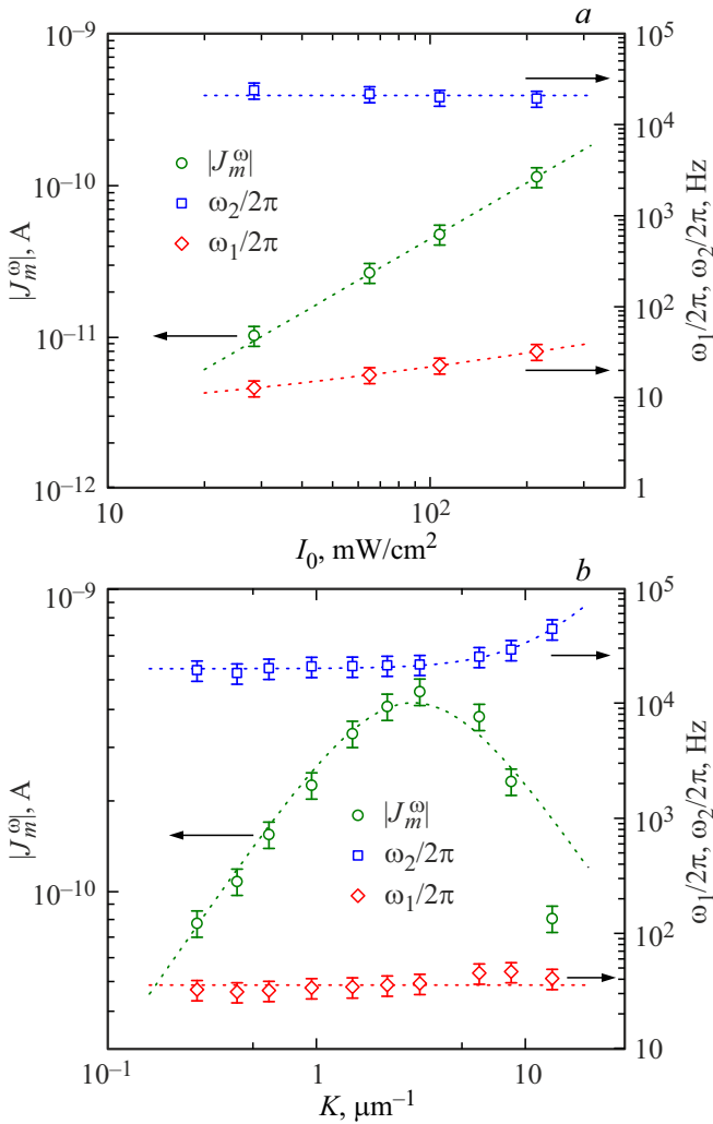
Рис. 2. a — зависимости максимальной амплитуды нестационарной фотоэдс и частот среза от средней интенсивности света при K = 0.42 \text{ мкм}^{-1} . b — зависимости максимальной амплитуды нестационарной фотоэдс и частот среза от пространственной частоты интерференционной картины при I_0 = 210 \text{ мВт/см}^2 .
