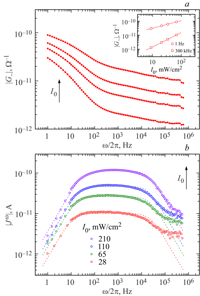
Рис. 1. a — частотные зависимости амплитуды отклика фотопроводимости на амплитудно-модулированный свет, снятые при различных средних интенсивностях света: I_0 = 9.0, 21, 34, 68 \text{ мВт/см}^2 . На вставке показаны зависимости |G_{\sim}|(I_0) для низкой и высокой частот модуляции. b — частотные зависимости амплитуды нестационарной фотоэдс при K = 0.42 \text{ мкм}^{-1} .
