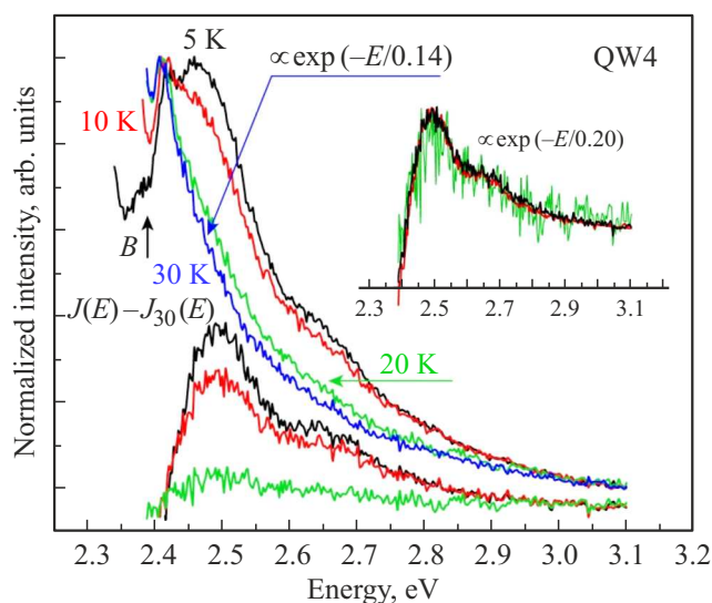
Рис. 3. Нормированные СВЛ слоя CdTe QW4 при различных температурах. В нижней части рисунка показано уменьшение вкладов носителей в формирование СВЛ при повышении температуры, на вставке эти вклады представлены в нормированном виде. J_{30} — форма СВЛ при T = 30 К. Вертикальной стрелкой указана энергия экситона барьерного слоя ZnTe.
