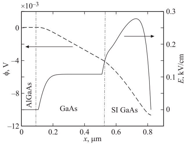
Рис. 7. Установившиеся распределения изменений потенциала и электрического поля с учетом динамики примесей.
