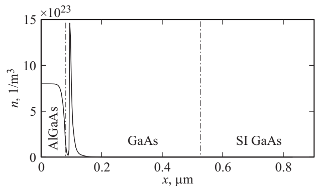
Рис. 2. Равновесное распределение концентрации электронов.
