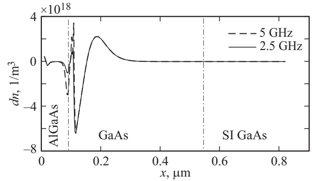
Рис. 4. Установившееся распределение изменения концентрации электронов в образце без учета динамики примесей.
