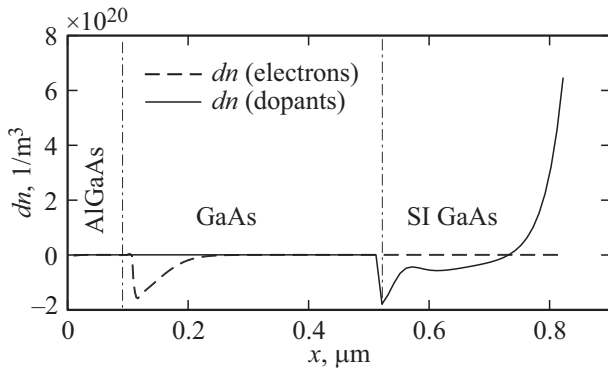
Рис. 6. Установившиеся распределения изменения концентраций электронов и примесей с учетом динамики примесей.
