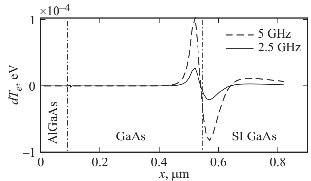
Рис. 5. Установившееся распределение изменения температуры электронного газа в образце без учета динамики примесей.
