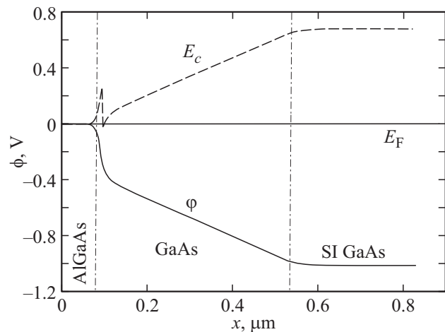
Рис. 3. Равновесное распределение потенциала ( \phi ) и края зоны проводимости ( E_c ). E_F — положение уровня Ферми.
