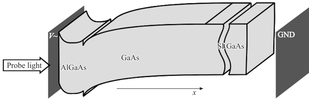
Рис. 1. Конфигурация гетероструктуры, которая исследовалась методом РМО.
