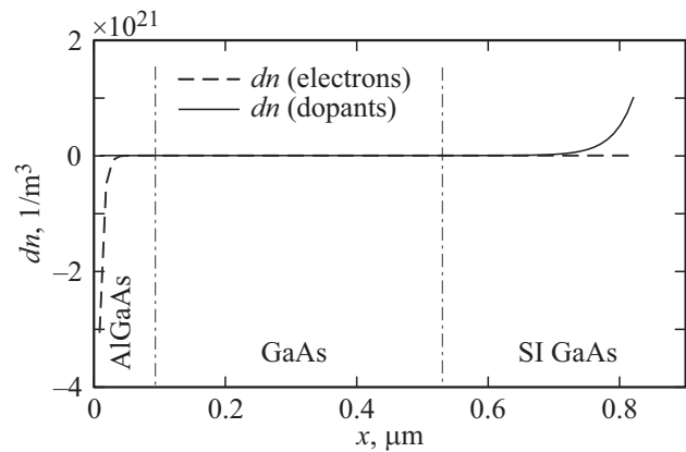
Рис. 9. Установившиеся распределения изменения концентраций электронов в зоне проводимости и на примесях при периоде электрического поля, много большем времени релаксации примесей.
