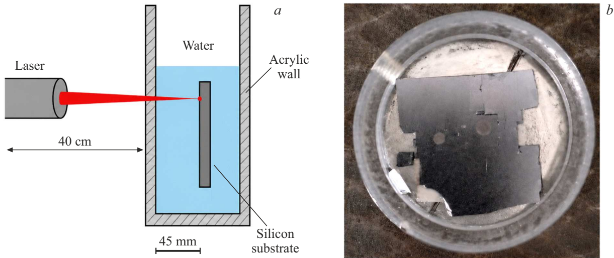
Рис. 1. a — схема установки генерации ударных волн; b — фотография кремниевой пластины.
