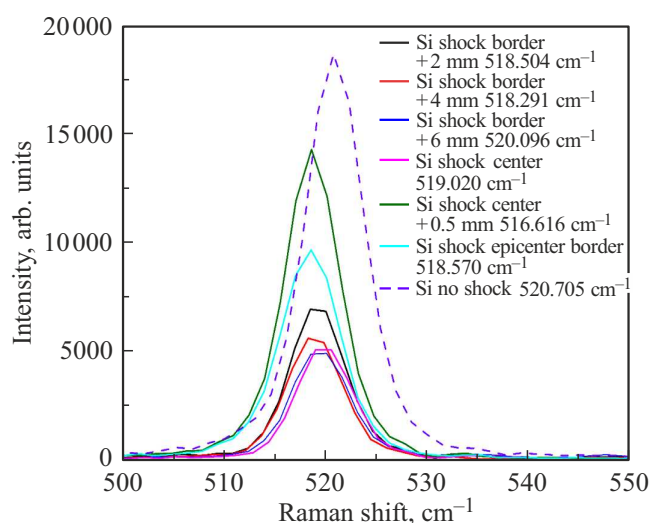
Рис. 2. Спектры КРС испытываемого образца.
