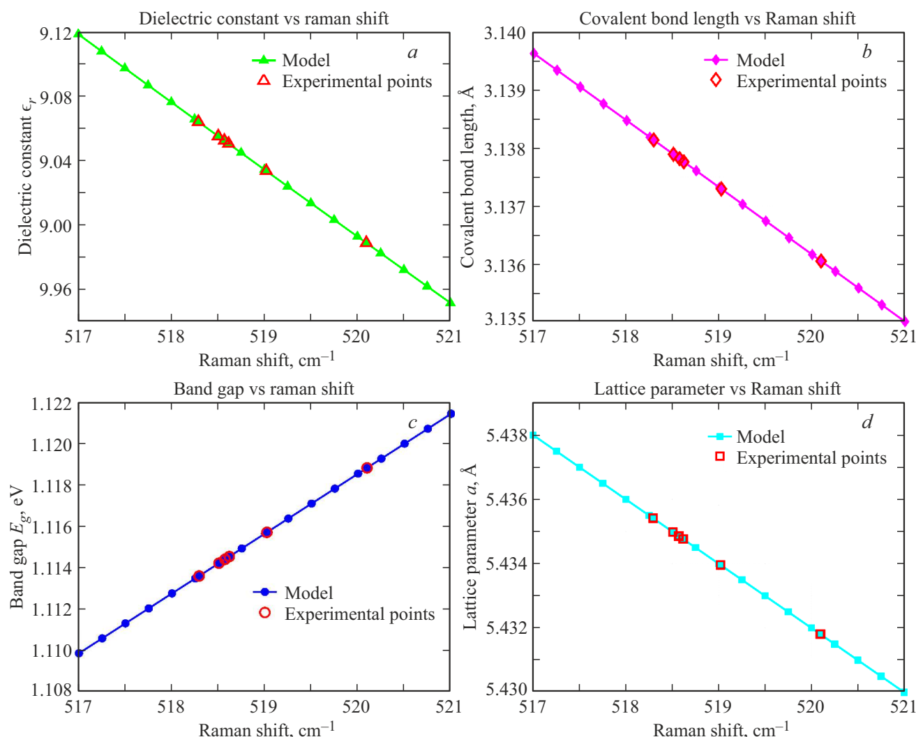
Рис. 3. Зависимость зонно-структурных параметров кремниевой пластины, подвергнутой ударно-волновой обработке, от наблюдаемого частотного сдвига спектра КРС: a — диэлектрической постоянной \epsilon(P) ; b — длины ковалентной связи d(P) ; c — ширины запрещенной зоны E_g(P) ; d — параметра кристаллической решетки a(P) .
