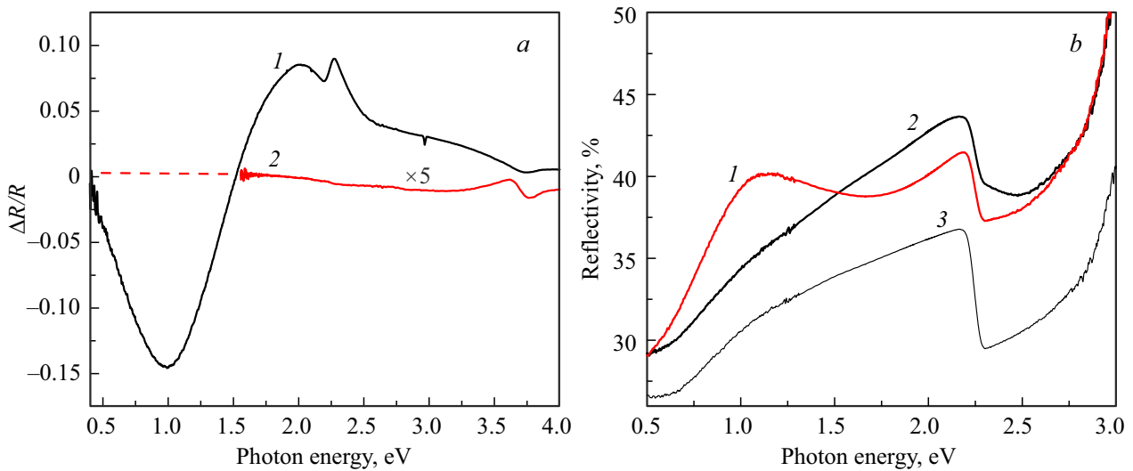
Рис. 2. a — измеренные спектры анизотропии отражения света \Delta R/R от поверхности (001) кристалла n -GaP с кластерами Au (1) и от поверхности n -GaP(001) без кластеров (2) (умножено на 5). b — коэффициенты нормального отражения от поверхности n -GaP света с поляризациями \alpha = y \parallel [110] (1) и с \alpha = x \parallel [110] (2) при наличии кластеров Au, а также R^{(0)} (3) в отсутствие кластеров.
