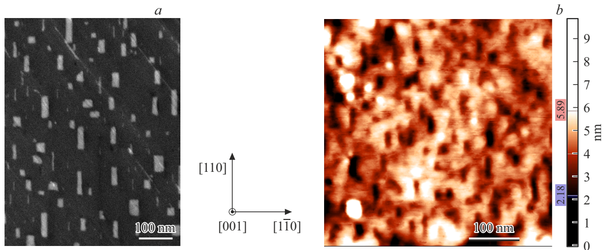
Рис. 1. a — СЭМ-изображение поверхности (001) кристалла GaP после отжига покрывающего слоя Au толщиной 10 нм в вакууме при температуре 400 °С в течение 30 мин. b — АСМ-изображение поверхности того же образца после химического удаления золота.
