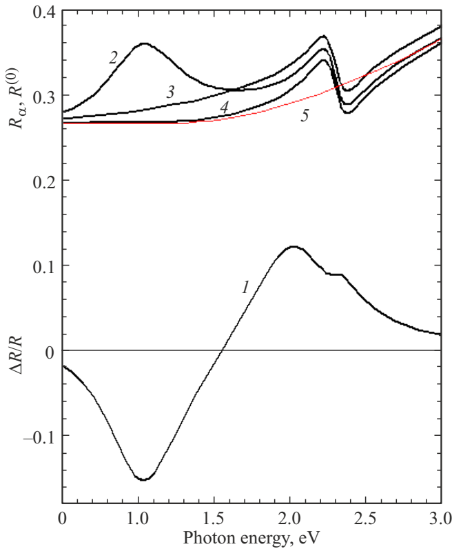
Рис. 3. Неоднородно уширенные спектры анизотропии отражения \Delta R/R (1) и поляризованного отражения R_y (2), R_x (3), рассчитанные по формулам (7)–(9) для структур Au/ n -GaP. Представлены также вычисленные спектры R^{(0)} нормального отражения света от кристаллов n -GaP (4) и p -GaP (5) в отсутствие кластеров. Использованы диэлектрические проницаемости GaP из работы [5] и Au из работы [7].
