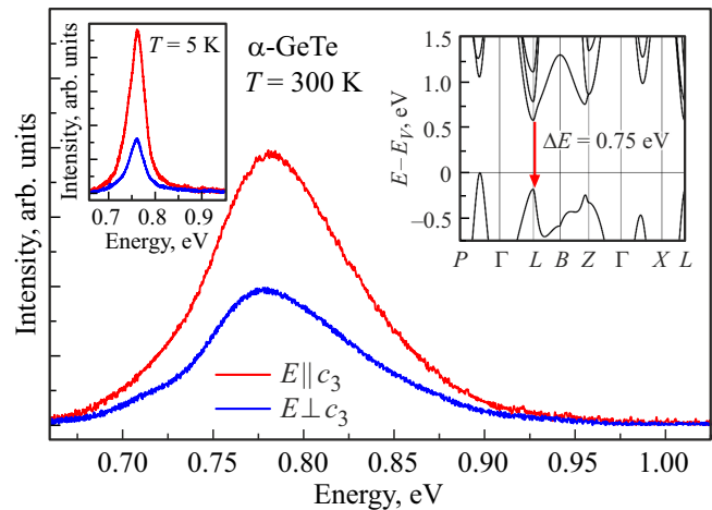
Рис. 3. Поляризованные спектры ФЛ образца \alpha\text{-GeTe} для грани (11\bar{2}0) , измеренные при T = 300 и 5 \text{ К} (левая вставка). Правая вставка — рассчитанная в работе электронная зонная структура \alpha\text{-GeTe} .
