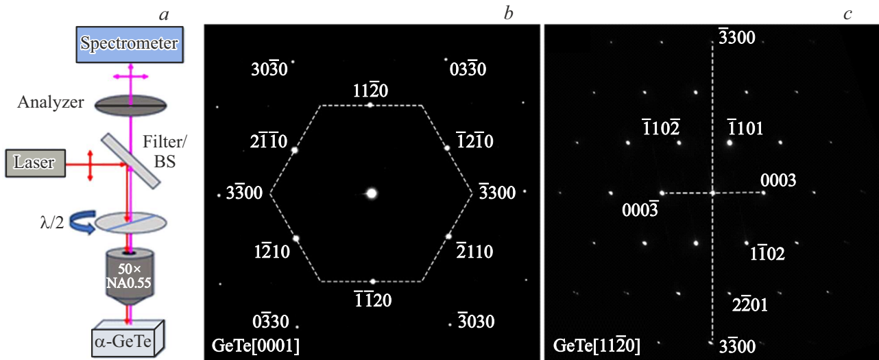
Рис. 1. a — схема эксперимента \mu -КРС с угловым разрешением; b и c — картины дифракции электронов для двух рассматриваемых в работе ориентаций кристаллов \alpha -GeTe на ПЭМ-сеточке: b — сечение кристалла по плоскости, близкой к базисной (0001); c — сечение по призматической плоскости типа 1120.
