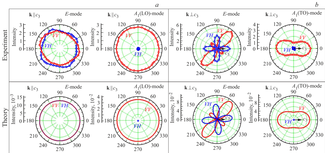
Рис. 2. Экспериментальные и теоретические полярные диаграммы зависимости интенсивности фоновых мод симметрии E и A_1(LO) в спектре КРС \alpha -GeTe. Геометрии эксперимента: a — волновой вектор \mathbf{k} излучения параллелен тригональной оси c_3 (сечение кристалла по плоскости, близкой к базисной (0001)); b — волновой вектор \mathbf{k} излучения перпендикулярен тригональной оси c_3 (сечение по призматической плоскости типа 1120).
