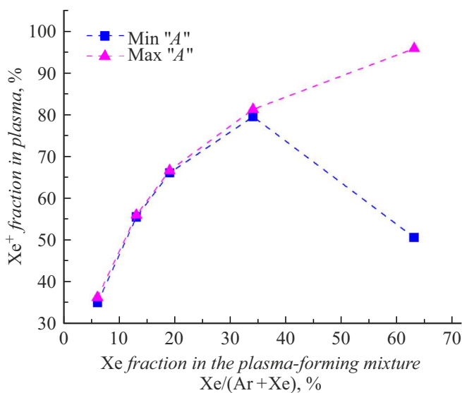
Рис. 3. Доля ионов Xe + в плазме при варьировании параметра A с сохранением требуемой T_e и n_e в зависимости от начальной доли Xe в плазмообразующей смеси при p = 10 \text{ mTorr} , W_{icp} = 1500 \text{ W} .
