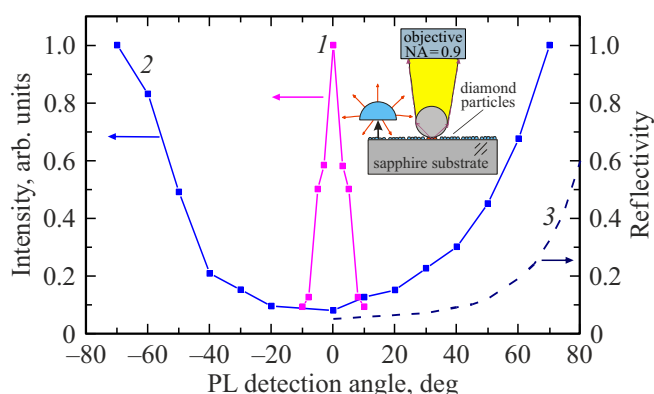
Рис. 2. Угловая зависимость интенсивности ФЛ БФЛ центра окраски SiV, полученная с применением стеклянной микросферы в схеме измерения ФЛ (1), без микросферы (2). Угловая зависимость коэффициента отражения от подложки сапфира (3). На вставке — схема эксперимента с микросферой. Алмазная частица на вставке выделена отдельной стрелкой в увеличенном масштабе.
