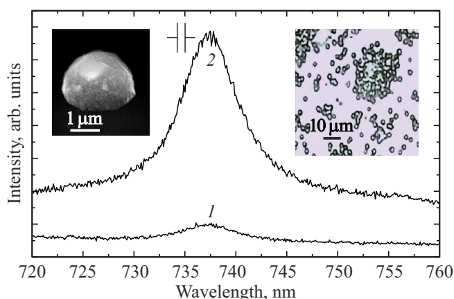
Рис. 1. Спектры ФЛ центра окраски SiV в алмазных микросферах, зарегистрированные без стеклянной микросферы перед микрообъективом (1), с микросферой (2). На вставках — изображение отдельной полусферической алмазной частицы, полученное с помощью растрового электронного микроскопа; изображение поверхности подложки с алмазными частицами, полученное с помощью оптического микроскопа.
