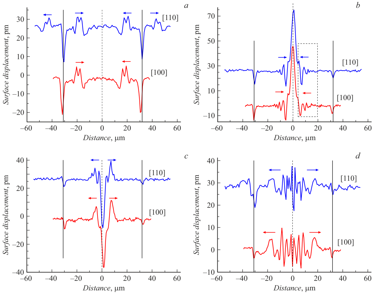
Рис. 2. Профили импульса ПАВ в моменты времени 1616 (а), 3056 (b), 3556 (c) и 4556 ps (d) вдоль направлений, эквивалентных {100} и {110}, показанных на рис. 1. Тонкие сплошные вертикальные линии обозначают область возбуждения, пунктирная вертикальная линия — примерное место фокуса. Стрелки указывают направление движения импульса ПАВ.
