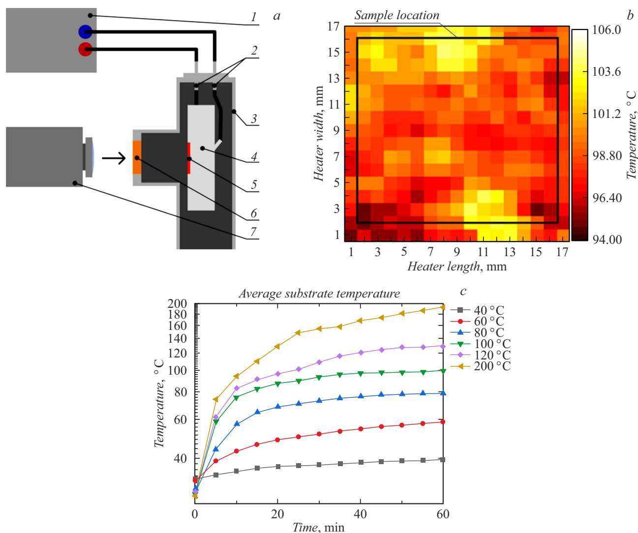
Рис. 3. a — принципиальная схема измерений температуры подложки: 1 — источник питания, 2 — тоководы, 3 — вакуумная камера, 4 — держатель образца, 5 — нагреватель, 6 — ZnSe стекло, 7 — тепловизор; b — распределение температуры по нагревателю подложки с указанной областью расположения образца; c — графики прогрева подложек.
