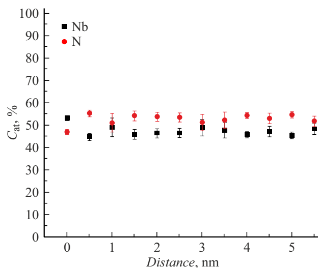
Рис. 6. Профиль распределения атомных концентраций элементов Nb и N по толщине пленки, измеренных методом EELS.
