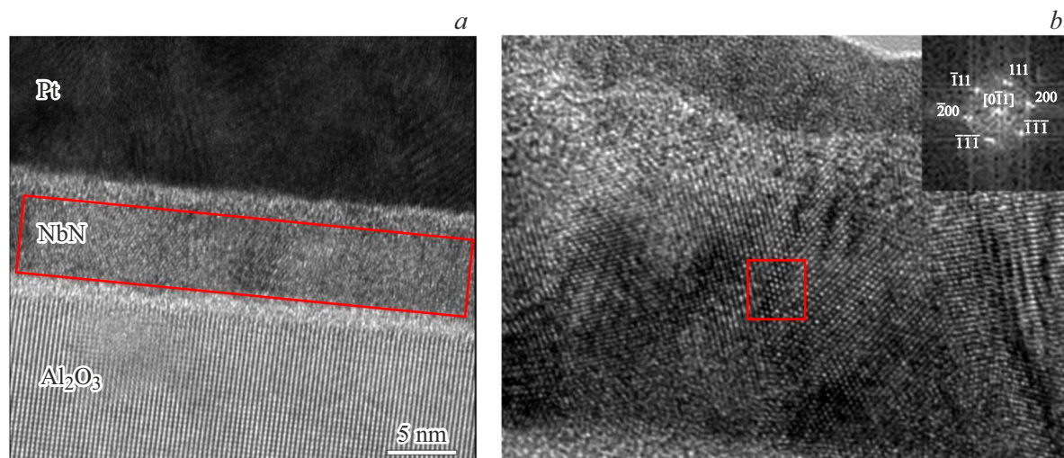
Рис. 7. Светлоскопическое ПЭМ изображение высокого разрешения поперечного среза образца поликристаллической пленки NbN на подложке из монокристаллического сапфира: а — общий вид; б — фазовый анализ, вставка — дифракция.
