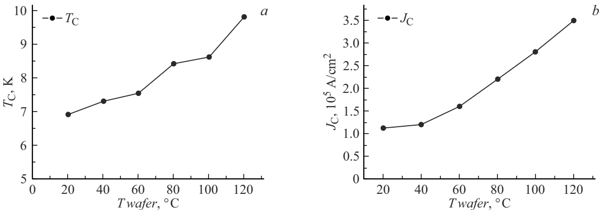
Рис. 5. Зависимости температуры перехода пленок в сверхпроводящее состояние из нормального T_C ( a ) и критической плотности тока J_C ( b ) от температуры подложки во время напыления.
