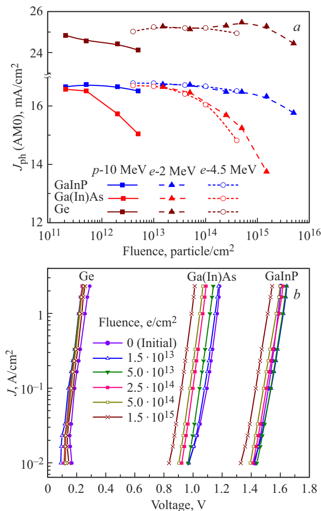
Рис. 1. Деградационные зависимости для плотностей фототоков субэлементов исследованных GaInP/Ga(In)As МП СЭ ( a ) до и после радиационного облучения 2 МэВ и 4.5 МэВ электронами и 10 МэВ протонами, а также зависимости „напряжение–ток“ для субэлементов, полученные методом электролюминесцентной диагностики при облучении 2 МэВ электронами ( b ). Зависимости „напряжение–ток“ при облучении 4.5 МэВ электронами и 10 МэВ протонами аналогичны представленным на рис. b и могут быть предоставлены по запросу.
