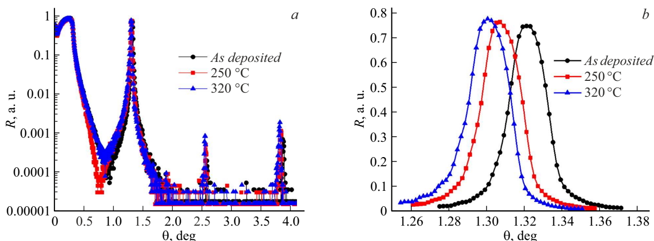
Рис. 6. Кривые зеркального отражения образца NiMo/C с d \approx 33.5 \text{ \AA} , синтезированного при C_{N_2} = 30\% и отожженного при 250 и 320 °C: a — общая кривая, b — первый порядок отражения.
