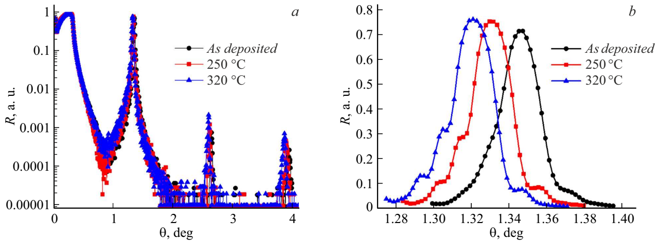
Рис. 4. Кривые зеркального отражения образца NiMo/C с d \approx 33.5 \text{ \AA} , синтезированного при C_{N_2} = 15\% и отожженного при 250 и 320 °C: a — общая кривая, b — первый порядок отражения.
