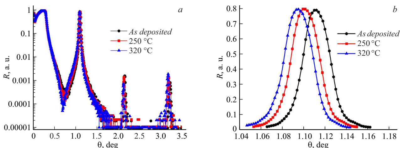
Рис. 5. Кривые зеркального отражения образца NiMo/C с d \approx 41.5 \text{ \AA} , синтезированного при C_{N_2} = 15\% и отожженного при 250 и 320 °C: a — общая кривая, b — первый порядок отражения.
