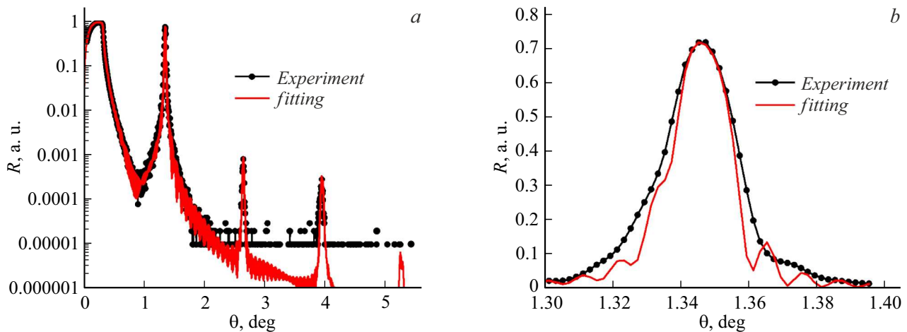
Рис. 3. Пример экспериментальной и смоделированной в „Multifitting“ кривых зеркального отражения образца NiMo/C с d \approx 33.5 \text{ \AA} : a — общая кривая, b — первый порядок отражения.
