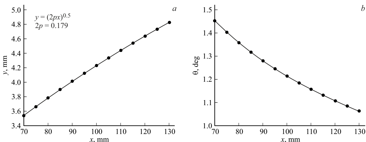
Рис. 2. Заданное уравнение направляющей параболического зеркала (а) и локальные углы скольжения излучения (b).
