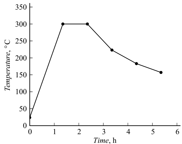
Рис. 1. Временная зависимость температуры образца многослойной структуры NiMo/C при нагреве до 300 °C.
