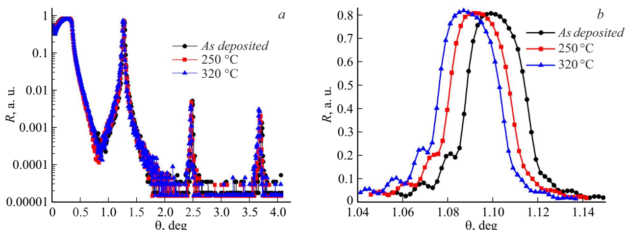
Рис. 7. Кривые зеркального отражения образца NiMo/C с d \approx 41.5 \text{ \AA} , синтезированного при C_{N_2} = 30\% и отожженного при 250 и 320 °C: a — общая кривая, b — первый порядок отражения.
