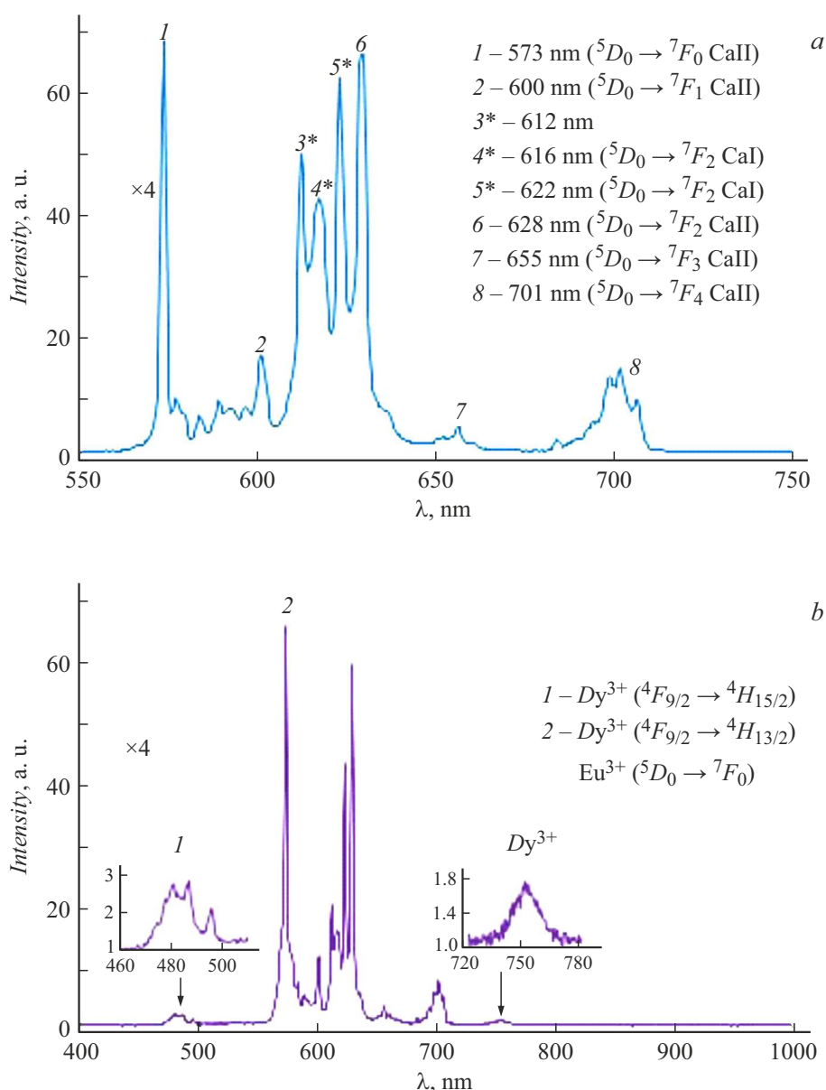
Рис. 1. a — фотолюминесценция ГАП:Eu, возбуждаемая св-лазером с \lambda = 405 nm (спектр увеличен в 4 раза). b — фотолюминесценция ГАП:Eu,Dy, возбуждаемая св-лазером с \lambda = 405 nm (спектр увеличен в 4 раза). Максимум 2 (573 nm) является суперпозицией максимумов 573 nm ( Eu^{3+} ) и 572 nm ( Dy^{3+} ). c — фотолюминесценция ГАП:Eu,B, возбуждаемая св-лазером с \lambda = 405 nm. d — фотолюминесценция ГАП:Eu,Y, возбуждаемая св-лазером с \lambda = 405 nm.
