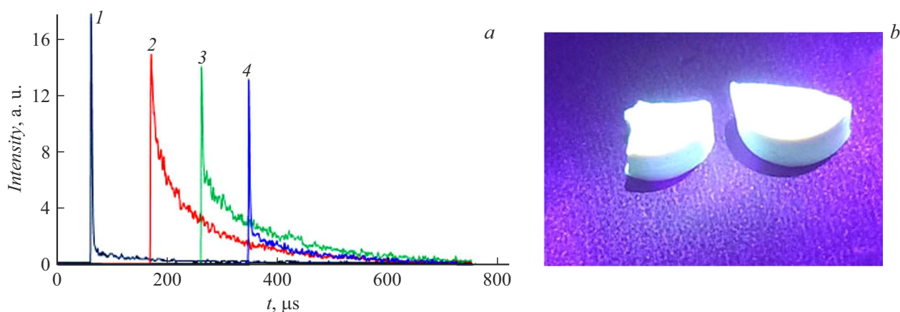
Рис. 2. a — кинетика затухания разных спектральных участков широкой полосы фотолюминесценции ГАП:Eu,Y при возбуждении лазерным излучением с длиной волны \lambda = 355 nm и длительностью импульса \tau = 8 ns. 1 — 520 nm (максимум полосы, обусловлен излучательными переходами ионов \text{Eu}^{2+} ), постоянная затухания \alpha \approx 1.6 \cdot 10^{-1} \mu\text{s}^{-1} , 2 — 573 nm (совпадает с максимумом излучательного перехода \text{Eu}^{3+} ( ^5D_0 \rightarrow ^7F_0 ), постоянная затухания \alpha \approx 1.4 \cdot 10^{-2} \mu\text{s}^{-1} . Кривые 3, 4 соответствуют окрестности перехода \text{Eu}^{3+} (573 nm), содержат быстро и медленно спадающие участки, обусловленные вкладом ионов \text{Eu}^{2+} и \text{Eu}^{3+} . b — изображение образца (таблетки) ГАП:Eu,Y при подсветке слабым излучением с \lambda = 405 nm.
