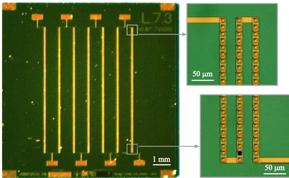
Рис. 1. Фотография массива джозефсоновских контактов Nb/NbSi/Nb. На вставках показаны фрагменты массива. Черным квадратом на нижней вставке обозначено положение одного из контактов.
