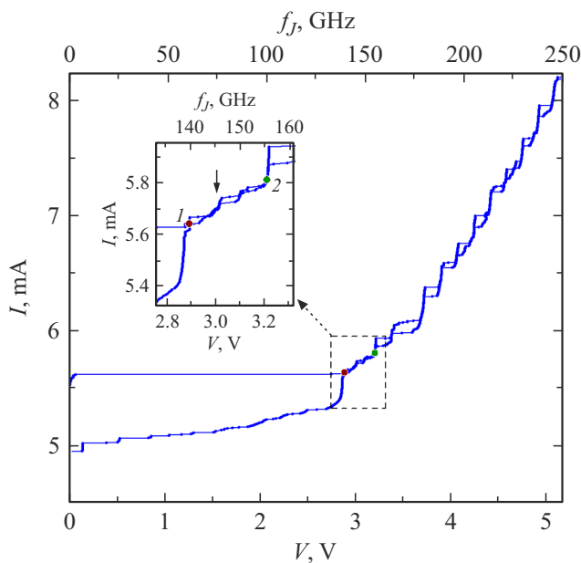
Рис. 2. ВАХ массива джозефсоновских контактов. На верхней оси отложена джозефсоновская частота, усредненная по всему массиву. В отмеченных на вставке точках проводились измерения, представленные на рис. 3. Стрелкой указана ступень, которой соответствует вторая спектральная линия на рис. 3, а.
