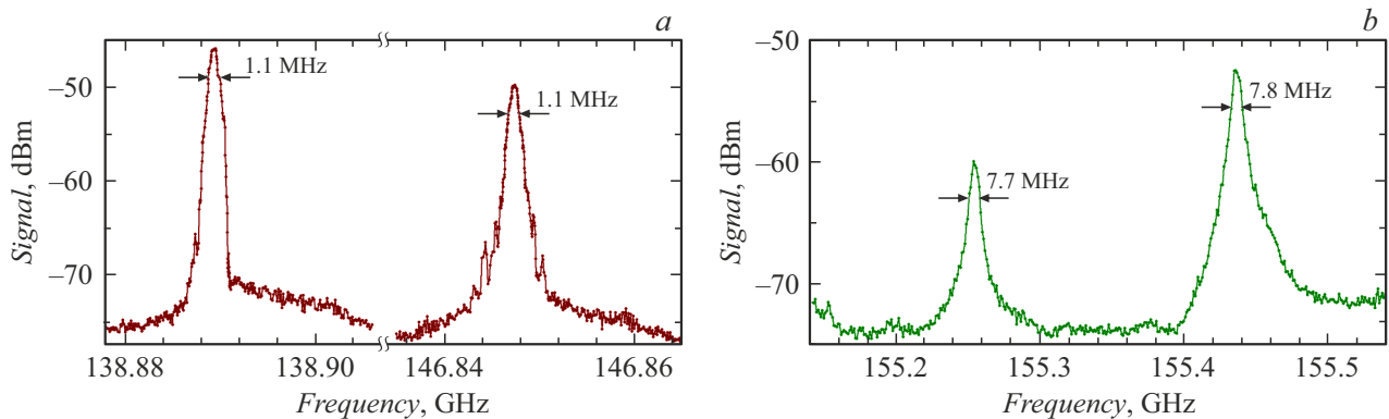
Рис. 3. Спектр джозефсоновской генерации, измеренный в точках ВАХ 1 (а) и 2 (б), отмеченных на рис. 2. Для каждой линии указана ширина, измеренная на уровне 1/2 от максимума.
