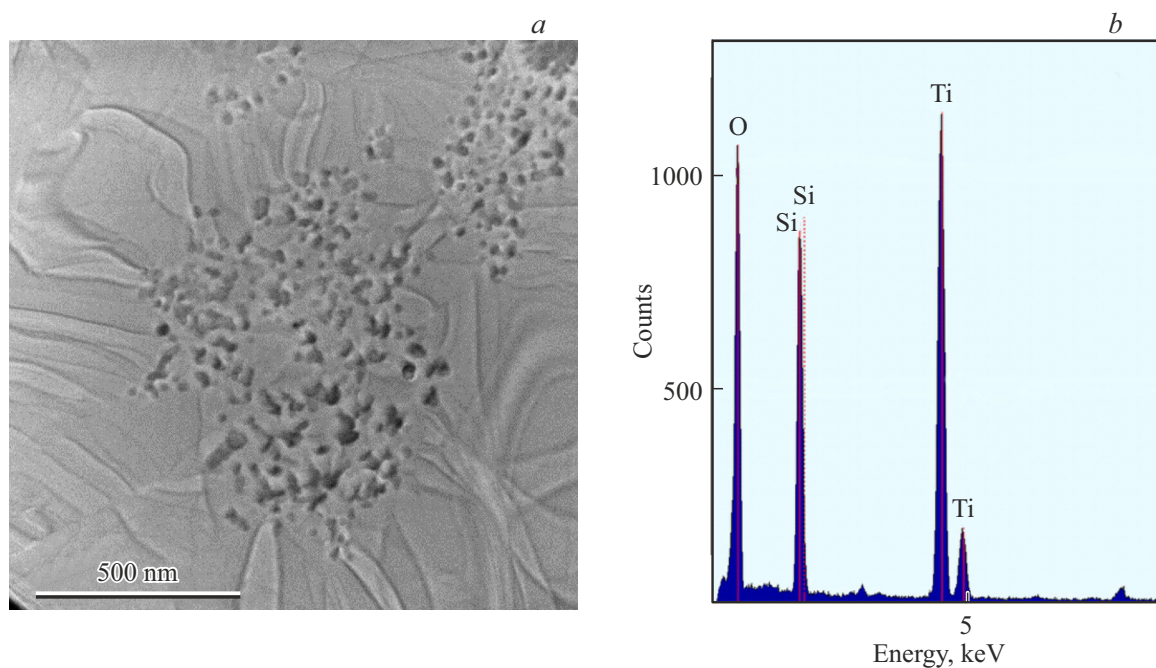
Рис. 2. ВРЭМ-изображение кристаллической структуры пленки стехиометрического состава \text{TiO}_2 после отжига при 973 К в течение 20 min в атмосфере аргона (а) и соответствующий EDX-спектр (b).
