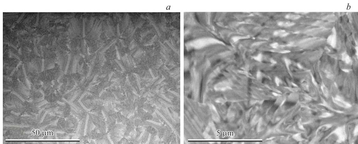
Рис. 1. СЭМ-изображения при разном увеличении кристаллической структуры пленки стехиометрического состава \text{TiO}_2 после отжига при температуре 973 К в течение 20 min в атмосфере аргона.
