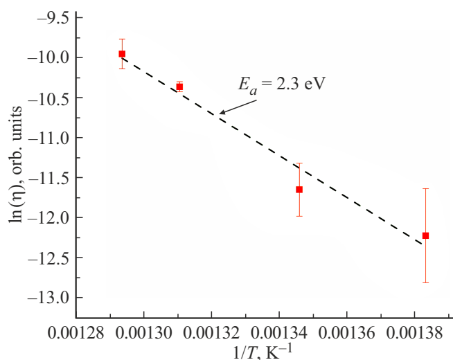
Рис. 8. Зависимость скорости фронта кристаллизации \eta от температуры отжига T . E_a — энергия активации движения фронта кристаллизации.
