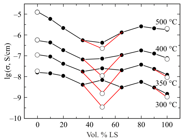
Рис. 6. Изотермы проводимости композитных пленок пироксидов \text{LaZrO}_{3.5} +перовскит \text{LaScO}_3 во влажном (темные кружки) и в сухом (светлые кружки) воздухе.
