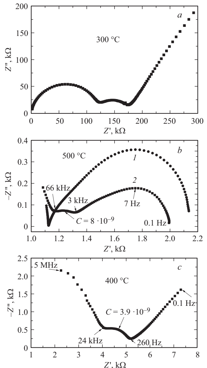
Рис. 3. Импедансные спектры ячеек \text{Ag}|f|\text{YSZ}|f|\text{Ag} : a ) с пленкой LS при 300^\circ\text{C} ; b ) без пленки (1) и с пленкой LS (2) при 500^\circ\text{C} ; c ) с пленкой LZ при температуре 400^\circ\text{C} .
