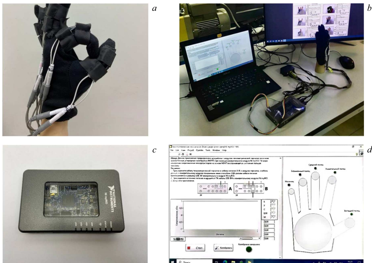
Рис. 6. Сенсорная интеллектуальная система распознавания жестов руки: a — неподвижные нанокompозитные тензорезистивные элементы на руке в области подвижных суставов пальцев в виде перчатки; b — интеллектуальная система распознавания жестов, состоящая из перчатки с нанокompозитными тензорезистивными элементами и измерительного модуля; c — внешний вид измерительного модуля; d — интерфейс приложения для считывания и хранения данных с нанокompозитных тензорезистивных элементов.
