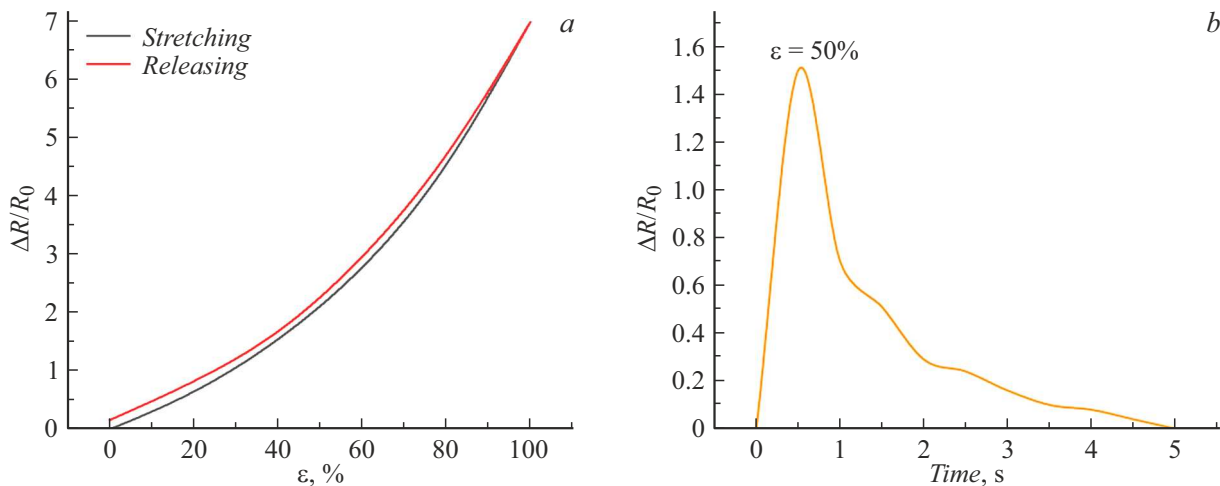
Рис. 4. Зависимость относительного изменения сопротивления при растяжении и релаксации (a); скорость восстановления активного слоя при 50% растяжении (b).
