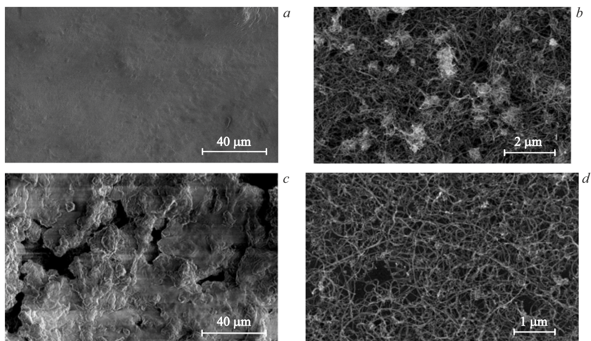
Рис. 2. СЭМ изображения активного слоя композитного тензорезистивного элемента на основе MWCNT и силикона без лазерного структурирования при различном увеличении ( a, b ) и с лазерным структурированием ( c, d ).
