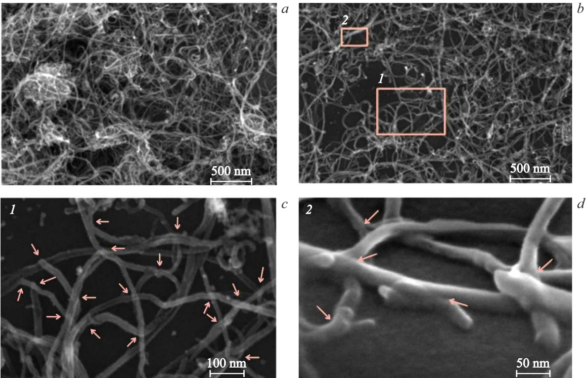
Рис. 3. Внутренняя структура активного слоя композитного тензорезистивного элемента, изготовленного без лазерного структурирования (а) и с лазерным структурированием (b–d). Изображение области 2 получено под углом 52°. Стрелками указаны сваренные участки нанотрубок, образованные в результате лазерного структурирования.
