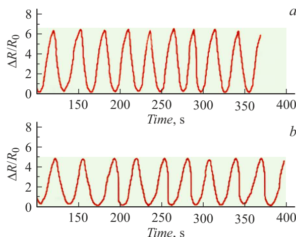
Рис. 9. Временные зависимости изменения относительного сопротивления для каждого нанокompозитного элемента на правой ( a ) и левой ( b ) частях ВНЧС во время его движения (открытия/закрытия) без восковых шаблонов (полная адентия).
