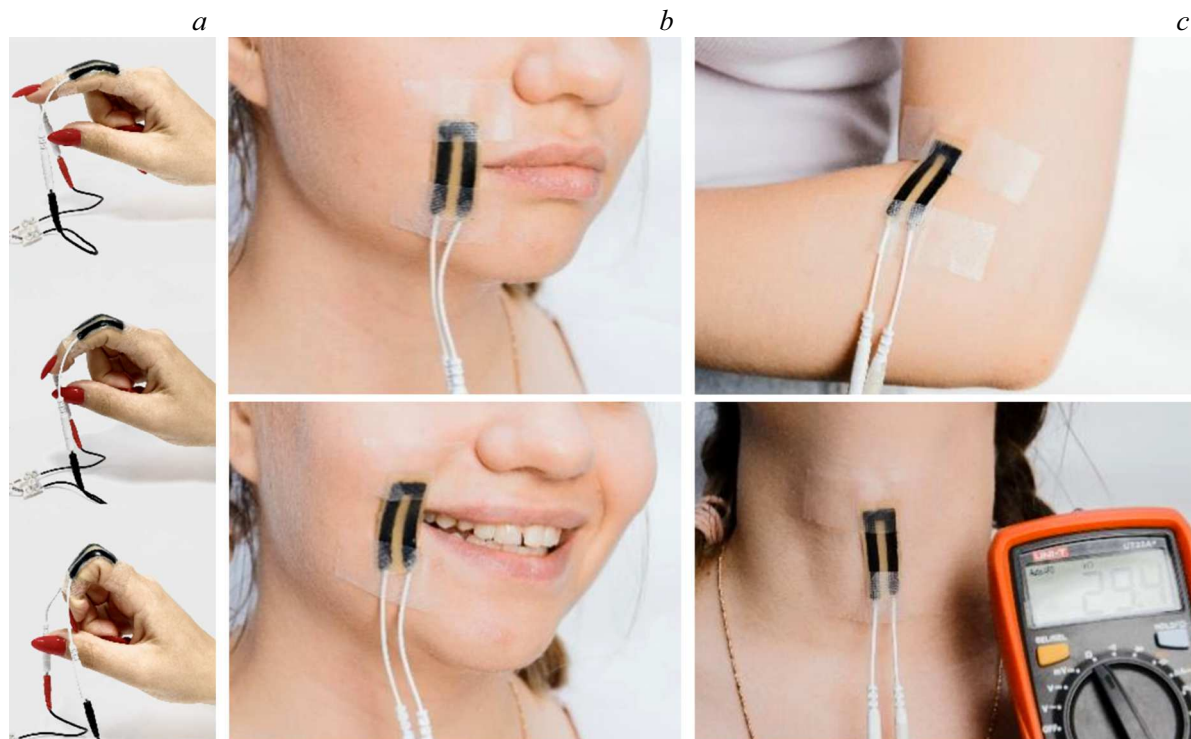
Рис. 5. Измерение деформации частей тела, вызванной анатомическими движениями: циклическая нагрузка на композитный тензорезистивный элемент при изгибе (a) пальца, (b) челюстно-лицевой области, (c) локтевого сустава и гортани.
