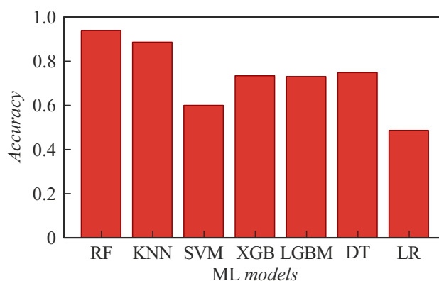
Рис. 7. Точность для следующих моделей машинного обучения: классификатор ближайших соседей (KNN), машина векторов поддержки (SVM), классификатор случайного леса (RF), классификатор xgboost (XGB), классификатор LightGBM (LGBM), классификатор дерева решений (DT), логистическая регрессия (LR) — при обучении на наборе данных размером 105 строк.
