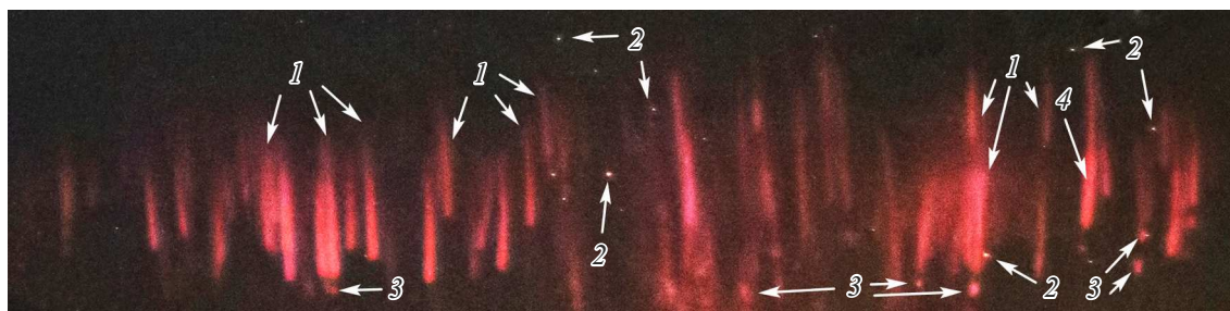
Рис. 9. Фотография столбчатых красных спрайтов, которая было получена исследователем ТСЯ, профессиональным фотографом, Frankie Lucena. Снимок был сделан 1 октября 2016 г. над областью грозовой активности в Cabo Rojo, Puerto Rico. 1 — столбчатые спрайты, 2 — наиболее яркие звезды, которые использовались для калибровки светимости красных спрайтов, 3 — яркие точки (beads), 4 — отдельные яркие области (glow).
