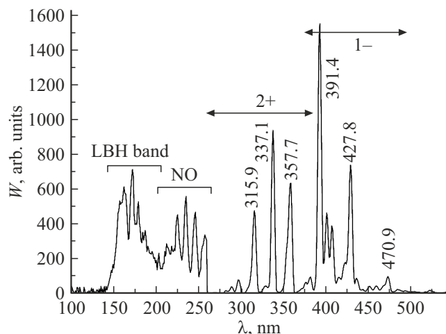
Рис. 3. Спектральная плотность энергии излучения W при разряде в воздухе из осевой части трубки. p = 0.35 Torr, f = 2 kHz. LBH — полосы Лаймана-Бирджа-Хопфилда. Интенсивность излучения в области 100–260 nm увеличена в 25 раз. Входная щель монохроматора 100 \mu\text{m} .
