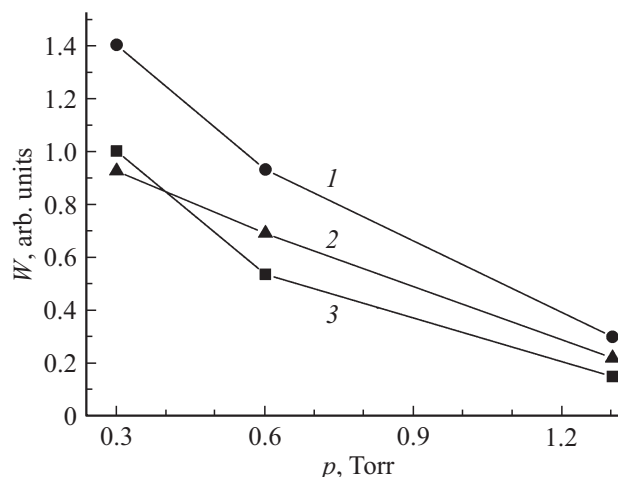
Рис. 5. Зависимости спектральной плотности энергии излучения W линии атомарного азота с длиной волны 174.3 нм от давления воздуха, полученные при положительной (1, 2) и отрицательной (3) полярностях высоковольтного электрода, при подключении высоковольтного вывода генератора к электроду 4 (1, 3) и к электроду 3 (2). Ширина щели монохроматора 25\ \mu\text{m} . f = 2 kHz.
