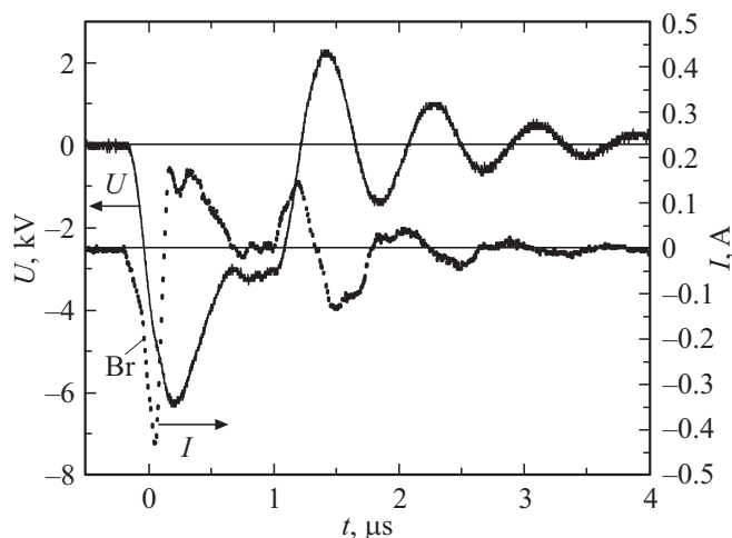
Рис. 2. Осциллограммы импульсов напряжения U между кольцевыми электродами и тока разряда I в цепи заземления генератора при давлении воздуха 0.6 Torr и f = 2 kHz.
