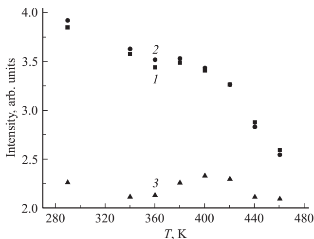
Рис. 2. Температурная зависимость интенсивности характерных полос на частотах 1110 (1) и 1490 \text{cm}^{-1} (2), а также фона на частоте 1330 \text{cm}^{-1} (3) в спектре КРС ДПВС.
