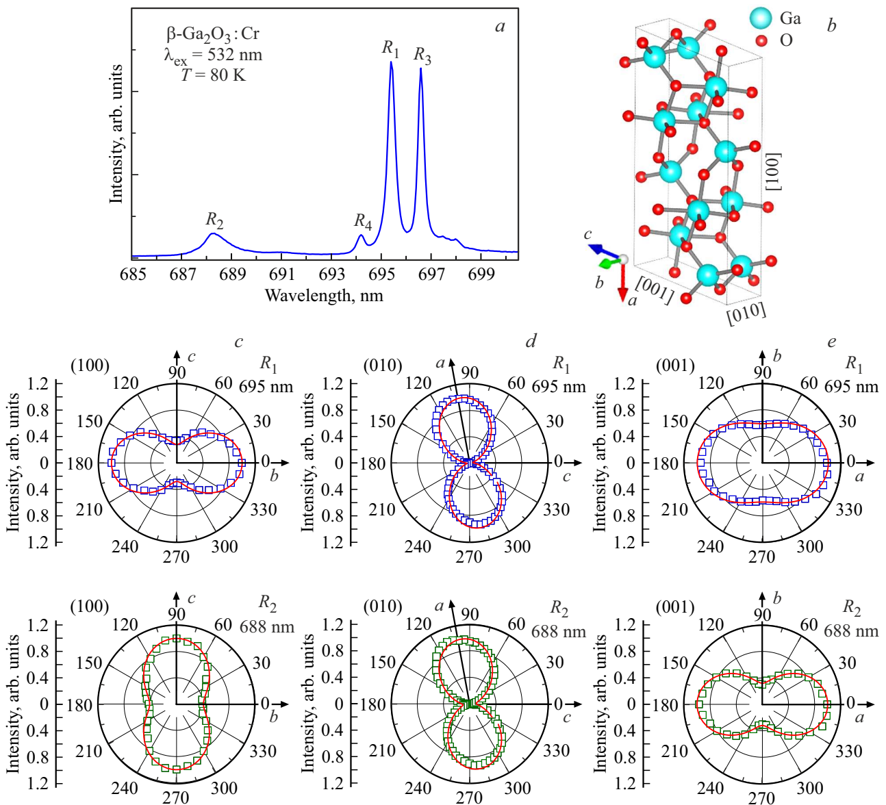
Рис. 1. a — Спектр ФЛ образца \beta\text{-Ga}_2\text{O}_3:\text{Cr} , полученный от плоскости (100); b — кристаллическая структура \beta\text{-Ga}_2\text{O}_3 ; c–e — зависимости интенсивности линий ФЛ R_1 и R_2 \beta\text{-Ga}_2\text{O}_3 , полученные от плоскостей (100) ( c ), (010) ( d ) и (001) ( e ), как функции угла между направлением вектора поляризации \mathbf{E} и кристаллографическими осями.
