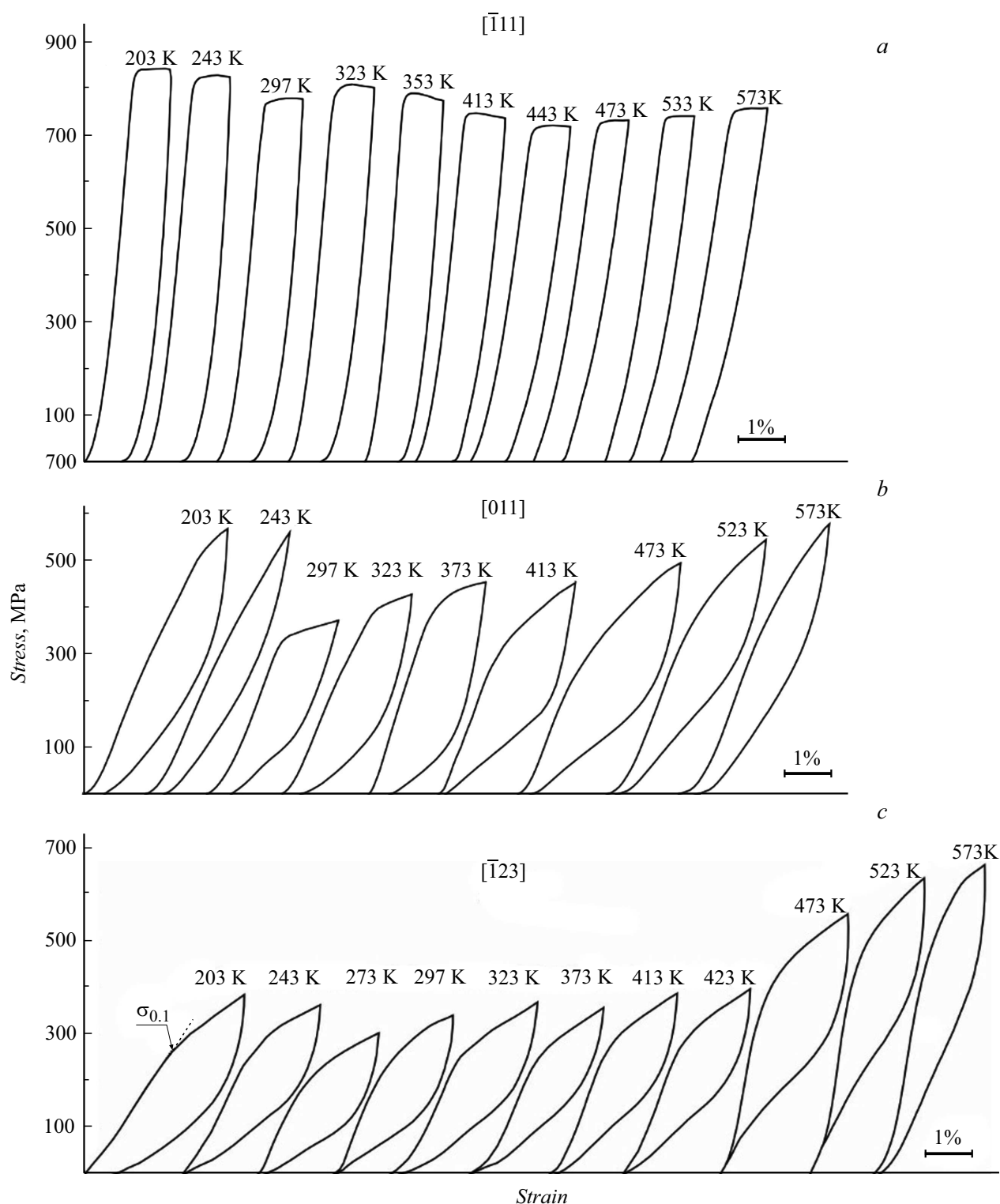
Рис. 1. Температурный интервал проявления эффекта сверхэластичности в монокристаллах сплава Fe–33Mn–11Al–7Ni–6Cr при сжатии. a — ориентация [111] , b — [011] , c — [123] .
