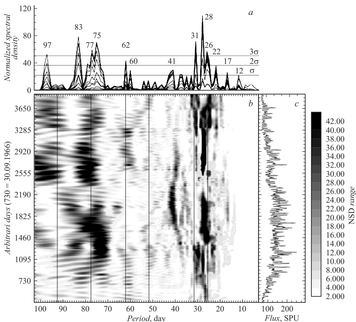
Рис. 2. a — CSP, b — NSD, вычисленные по значениям посуточного радиоиндекса ( c ) на интервале пробных периодов от 3 до 103 дней для 20-го цикла СА. NSD построена в скользящем временном окне шириной 731 день. По оси ординат диаграммы NSD отложены относительные дни, отсчитываемые от даты начала 20-го цикла — 01.10.1964. Три полосы, нанесенные на поле диаграммы справа налево, обозначают соответственно интервалы допустимых значений (от экватора ( 0^\circ ) до широты 45^\circ ) изменения периодов одинарного, двойного и тройного синодического оборота Солнца.
