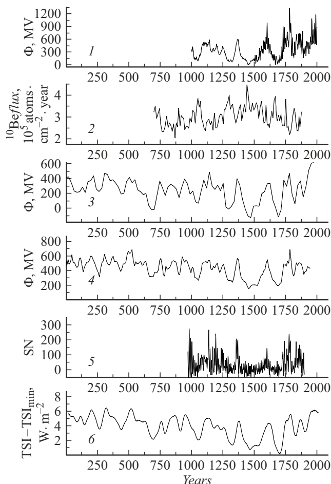
Рис. 1. Индикаторы солнечной активности, использованные в работе: 1 — солнечный модуляционный потенциал [4]; 2 — концентрация ^{10}\text{Be} во льду Антарктиды [5]; 3 — солнечный модуляционный потенциал [6]; 4 — солнечный модуляционный потенциал [7]; 5 — число солнечных пятен [8]; 6 — полная солнечная радиация [9].
