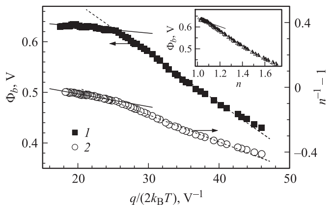
Рис. 2. Зависимости величин Φ b (кривая 1) и ( n -1 - 1) (2) от обратной температуры. На вставке — зависимость высоты барьера Шоттки от фактора неидеальности n . Точки — эксперимент, прямые — линейная аппроксимация в диапазонах 230–330 К (сплошные) и 120–220 К (штриховые).
