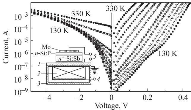
Рис. 1. Вольт-амперные характеристики диодов Шоттки Mo/ n-n + -Si в температурном диапазоне 130–330 К. Приведены кривые, измеренные с шагом 20 К. На вставке — схема ультразвукового нагружения образца: 1 — диэлектрический слой; 2 — пьезоэлектрический преобразователь LiNbO 3 ; 3 — экранирующий слой; 4, 5 — электроды для возбуждения ультразвука и измерения вольт-амперной характеристики соответственно. Суммарная толщина диэлектрического и экранирующего слоев 0.02 мм.
