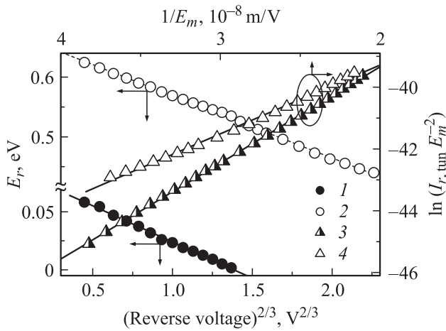
Рис. 4. Полевые зависимости характеристической энергии (кривые 1, 2) и независящей от температуры компоненты обратного тока в координатах Фаулера–Нордгейма (3, 4) при T = 120–220 К (1, 3) и T = 230–330 К (2, 4). Точки — эксперимент, прямые — линейная аппроксимация.
