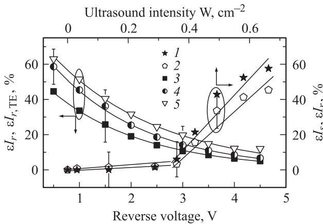
Рис. 5. Зависимости относительных акустоиндуцированных изменений тока насыщения (кривая 1) и обратного тока при V_r = 1 В (2) от интенсивности ультразвукового нагружения, а также зависимости относительных акустоиндуцированных изменений обратного тока (3, 4) и относительного вклада ТЭ слагаемого в общий обратный ток (5) от обратного смещения. W_{us} , Вт/см 2 : 3 — 0.49, 4 — 0.66, 5 — 0. f_{us} = 9.6 МГц, T = 296 К.
