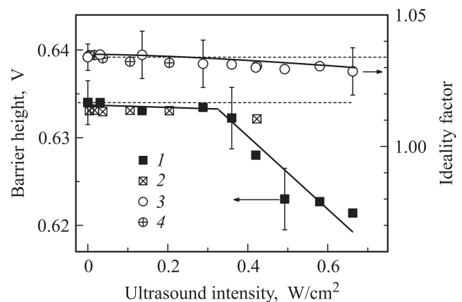
Рис. 3. Зависимости высоты барьера Шоттки (кривые 1, 2) и фактора неидеальности (3, 4) от интенсивности ультразвукового нагружения при T = 296 К. f_{us} , МГц: 1, 3 — 9.6, 2, 4 — 30.1. Горизонтальные штриховые линии — значения параметров при отсутствии ультразвукового нагружения.
