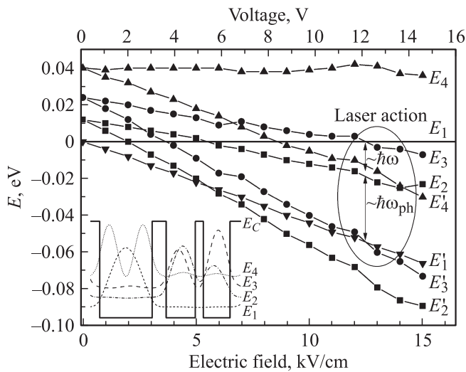
Рис. 2. Зависимость взаимного положения электронных уровней энергии в двух соседних каскадах гетероструктуры ККЛ-2 от приложенного электрического поля ( E_i — энергии в первом, E'_i — в следующем каскаде, энергии отсчитываются от уровня E_1 ); на вставке — зонная диаграмма и квадраты волновых функций электронов при нулевом поле.
