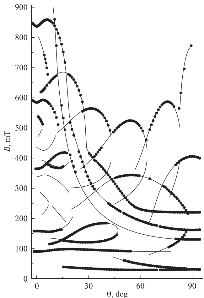
Рис. 3. Полярная угловая зависимость положений переходов тригональных центров Gd^{3+} в ромбоэдрической фазе (образец ЧМ), точки — эксперимент, кривые — расчет с параметрами спинового гамильтониана [5].
