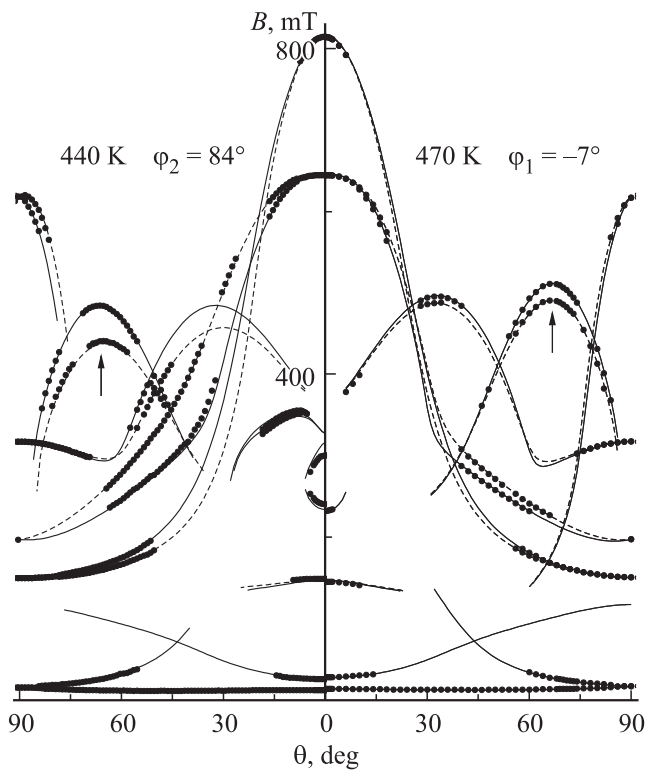
Рис. 4. Полярные угловые зависимости положений переходов тригональных центров Fe^{3+} ромбоэдрической фазы (образец ЧМ) в двух ортогональных плоскостях. Точки — эксперимент при 440 и 470 К, сплошные и штриховые кривые — расчет с параметрами (2) для двух МНЭ-центров при указанных углах \varphi . Стрелками помечены переходы между уровнями энергии 4 \leftrightarrow 5 (нумерация снизу).
