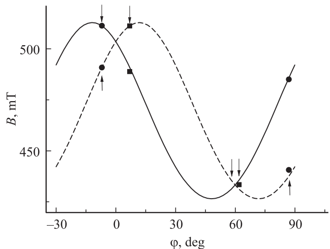
Рис. 5. Расчетная азимутальная зависимость положений переходов 4 \leftrightarrow 5 МНЭ-центров при \theta = 66^\circ (см. рис. 4) с параметрами (2), штриховая кривая — c_{43} > 0 , сплошная — c_{43} < 0 . Нижними стрелками отмечены азимутальные углы, при которых проведены измерения на образце (ЧМ), верхними — углы, реализовавшиеся в блоках образца (БЗПМ), точки — экспериментальные положения сигналов данного перехода.
