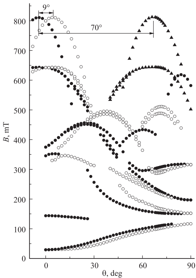
Рис. 2. Ориентационное поведение переходов центров Fe^{3+} в образце (БЗПМ) в ромбоэдрической фазе приблизительно в плоскости C_3-C_3 двух доменов. Расщепление сигналов при произвольных углах \theta обусловлено наличием двух магнитно неэквивалентных центров. Положения сигналов в блоках, оси C_3 которых развернуты на \approx 9^\circ , представлены черными и белыми точками соответственно, треугольниками — положения переходов во втором домене.
