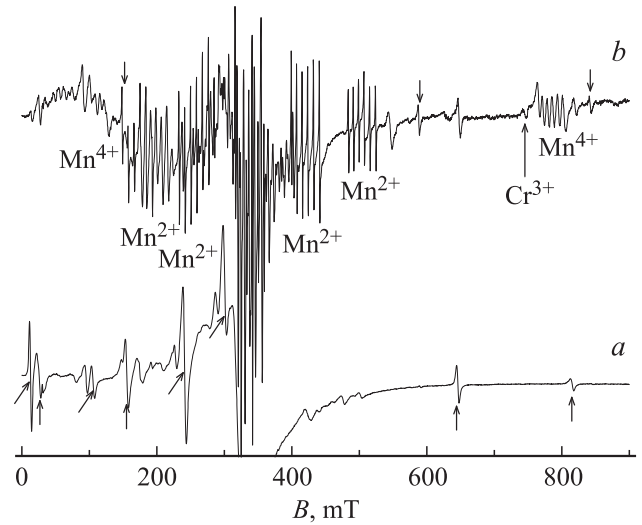
Рис. 1. ЭПР-спектр (первая производная спектра поглощения) галлата лантана с примесью 2% Mn в ромбоэдрической фазе при \mathbf{B} \parallel C_3 , где \mathbf{B} — индукция магнитного поля. (a) — образец, выращенный методом зонной плавки, (b) — методом Чохральского. Верхние стрелки — переходы центров \text{Gd}^{3+} в домене с C_3 \parallel B , нижние стрелки — переходы ионов \text{Fe}^{3+} в домене с C_3 \parallel B , наклонные стрелки — переходы ионов \text{Fe}^{3+} в доменах с \theta = 70,5^\circ .
