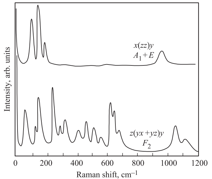
Рис. 2. Спектры Pr_3Sb_5O_{12} при x(zz)y и z(yx + yz)y геометриях рассеяния.
