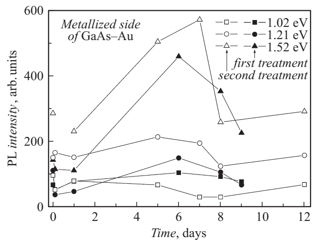
Рис. 2. Зависимости интенсивности полос ФЛ Au-GaAs от времени выдержки образцов.
