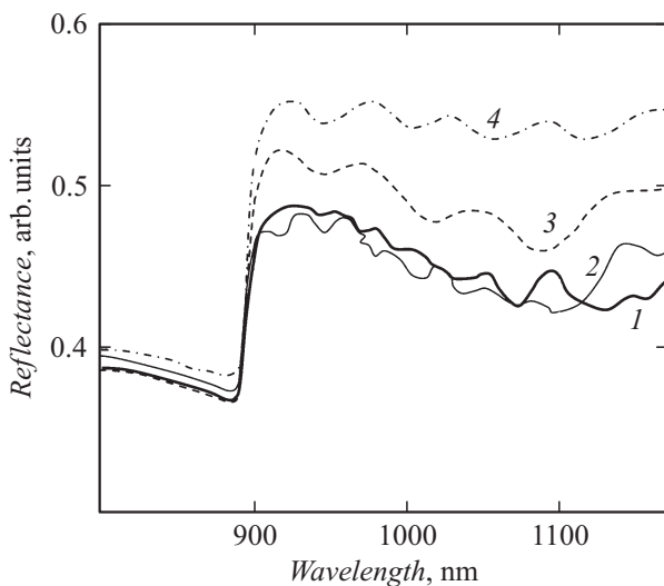
Рис. 1. Спектры оптического отражения эпитаксиальных структур n-n^+ арсенида галлия до и после микроволновой обработки: 1 — исходный, 2 — сразу после СВЧ-обработки, 3 — через 30 min, 4 — через 1.5 h после обработки и через 24 h.
